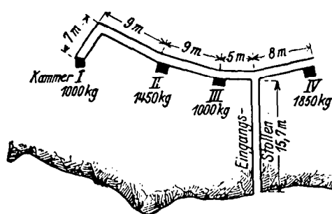
Lageplan 1:250
